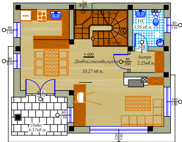
РАЗПРЕДЕЛЕНИЕ НА ПЪРВИ ЕТАЖ М 1:50 Площ на етажа 63.88 кв.м.
