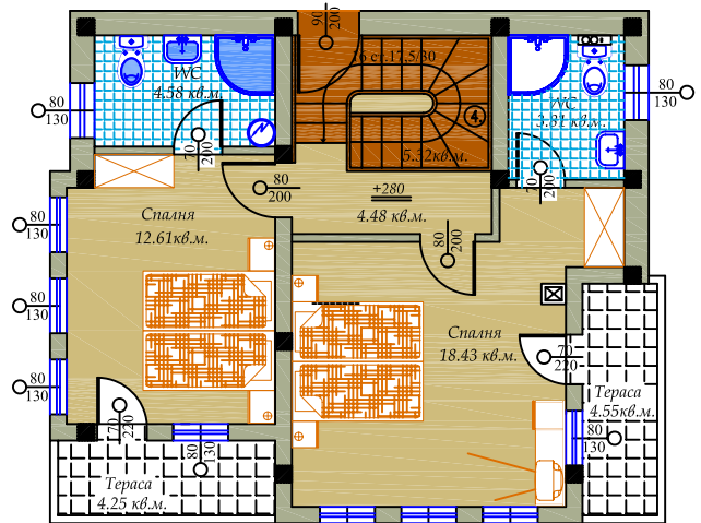
РАЗПРЕДЕЛЕНИЕ НА ВТОРИ ЖИЛ. ЕТАЖ М 1:50 Площ на етажа 70.17 кв.м.
