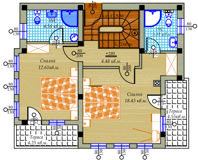
РАЗПРЕДЕЛЕНИЕ НА ВТОРИ ЖИЛ. ЕТАЖ М 1:50
