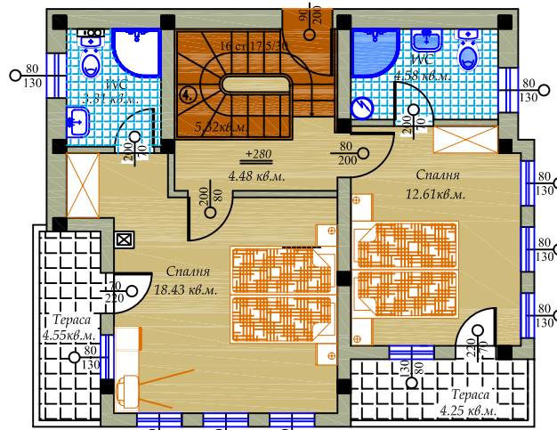
РАЗПРЕДЕЛЕНИЕ НА ВТОРИ ЖИЛ. ЕТАЖ М 1:50
