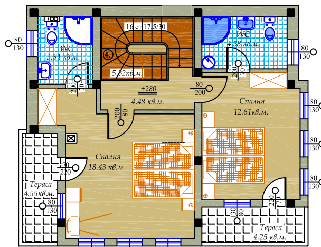
РАЗПРЕДЕЛЕНИЕ НА ВТОРИ ЖИЛ. ЕТАЖ М 1:50
