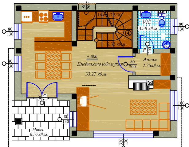
РАЗПРЕДЕЛЕНИЕ НА ПЪРВИ ЕТАЖ М 1:50
