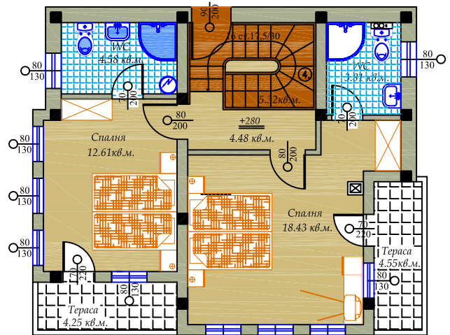
РАЗПРЕДЕЛЕНИЕ НА ВТОРИ ЖИЛ. ЕТАЖ М 1:50
